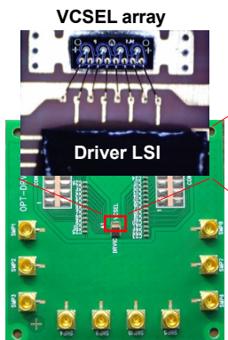
10-Gb/s VCSEL ドライバLSI 90-nm CMOS
