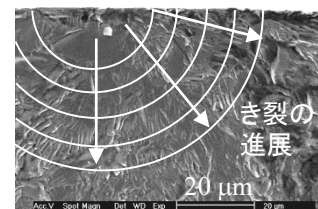
図4 高強度で疲労強度が低下するマルエージング鋼で発生する脆性型のき裂
